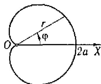
28. Кардиоида
