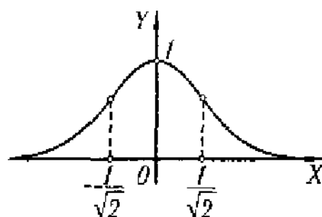
16. Кривая Гаусса y = e^{-x^2} .
