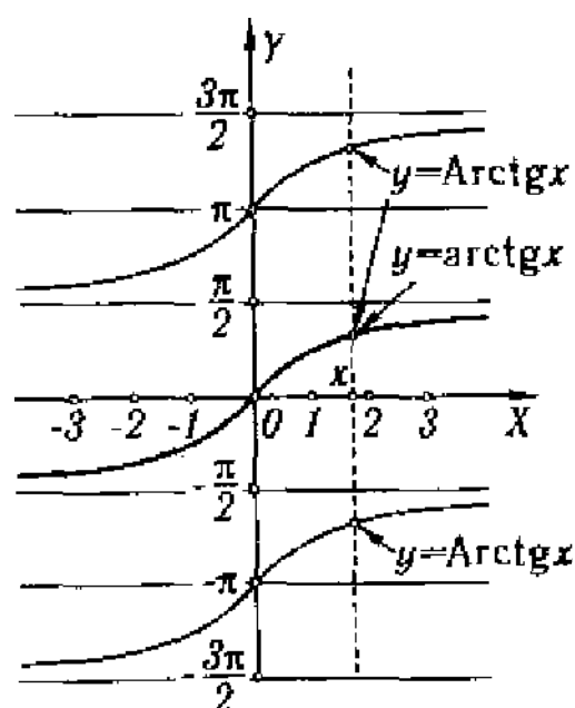
13. Графики обратных тригонометрических функций y = \text{Arctg } x и y = \text{Arctg } x .
