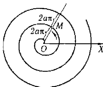
30. Спираль Архимеда r = a\varphi ( r \geq 0 ).
