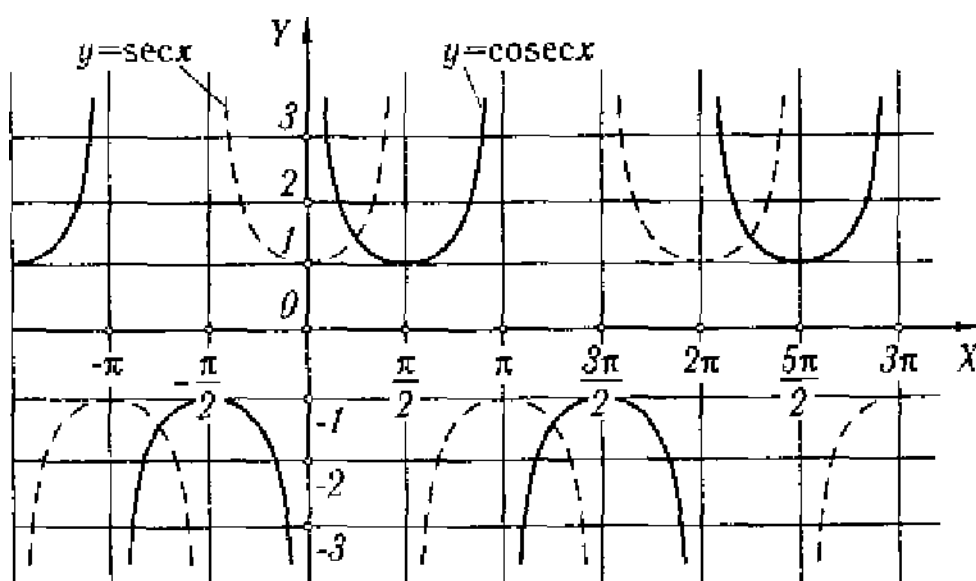
11. Графики функций y = \sec x и y = \operatorname{cosec} x .
