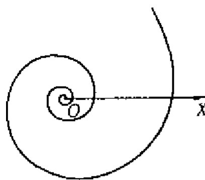
33. Логарифмическая спираль
