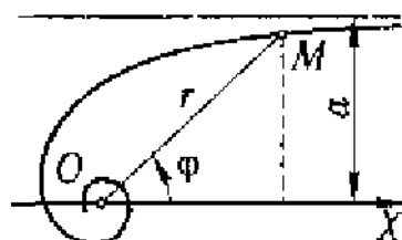
32. Гиперболическая спираль
