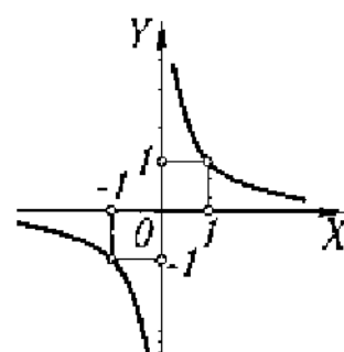
3. Равноосная гипербола y = \frac{1}{x} .
