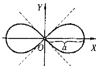
25. Лемниската Бернулли
