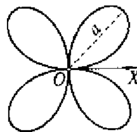
34. Четырехлепестковая роза r = a |\sin 2\varphi|.
